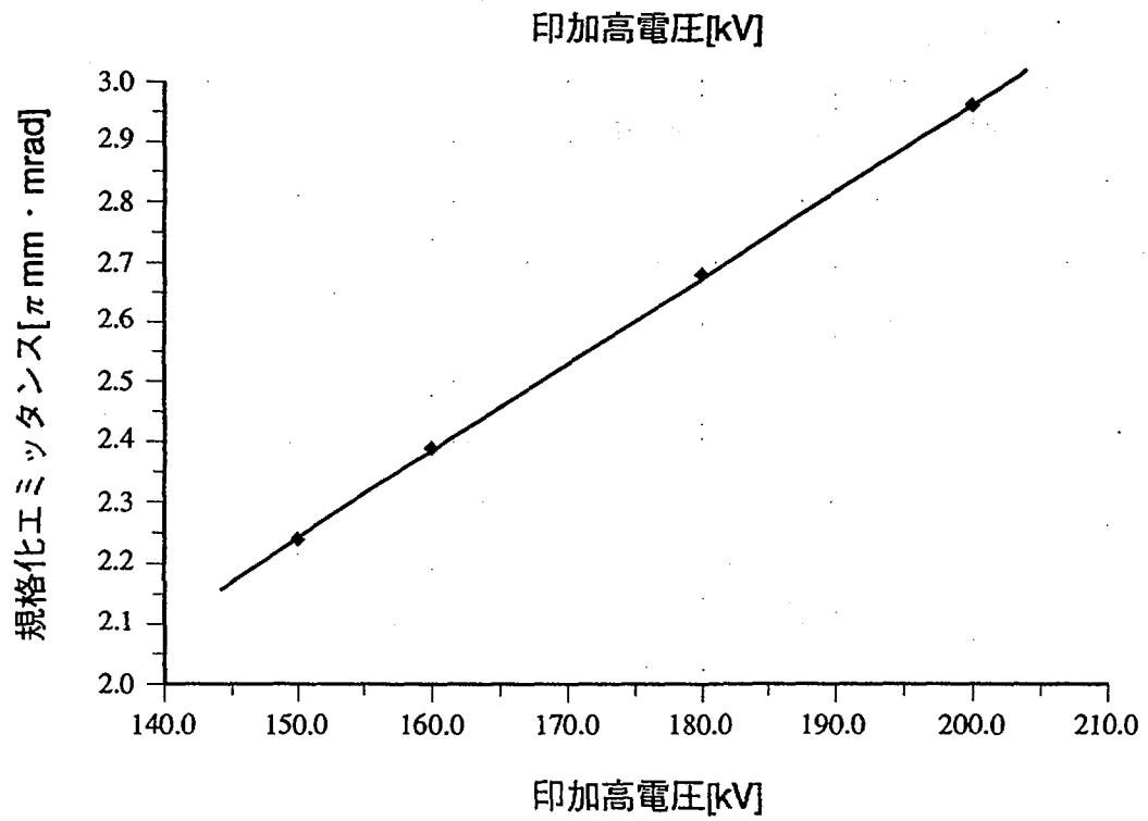
図 8 EGUNによる数値計算結果
