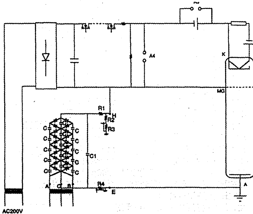
図1 電子銃の電源回路系統
