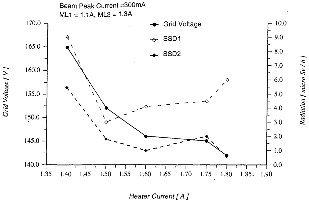
図17 電流値300mA、HV180kVのときのヒーター電流、グリッド電圧の最適値の測定
