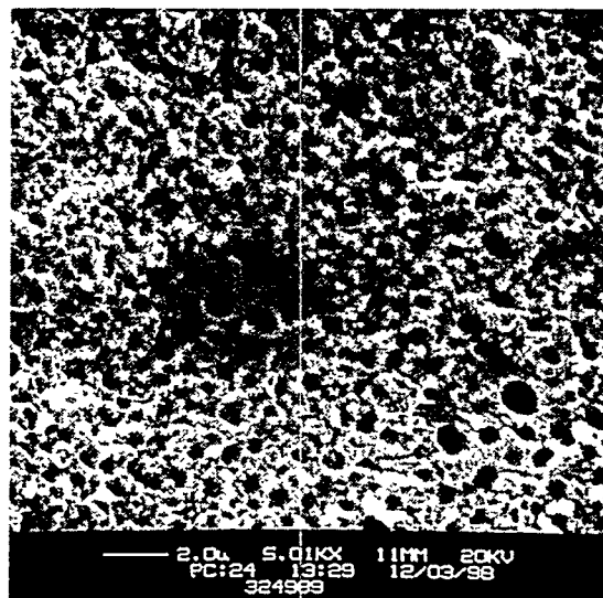
(d) U-6Mo-1Pt
