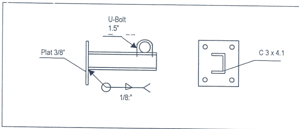
Gambar 4. Skets penyangga pipa lurus.
