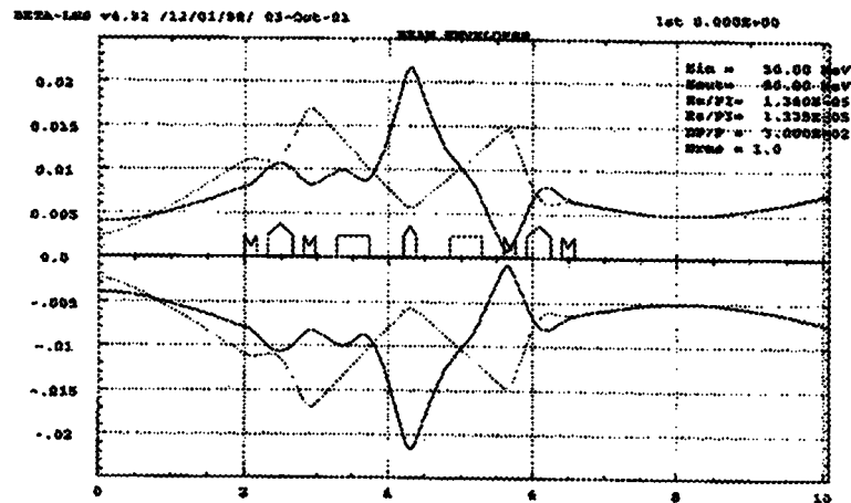
Fig.5 : Enveloppes du faisceau pour le cas : aimant secteur sans indice.
