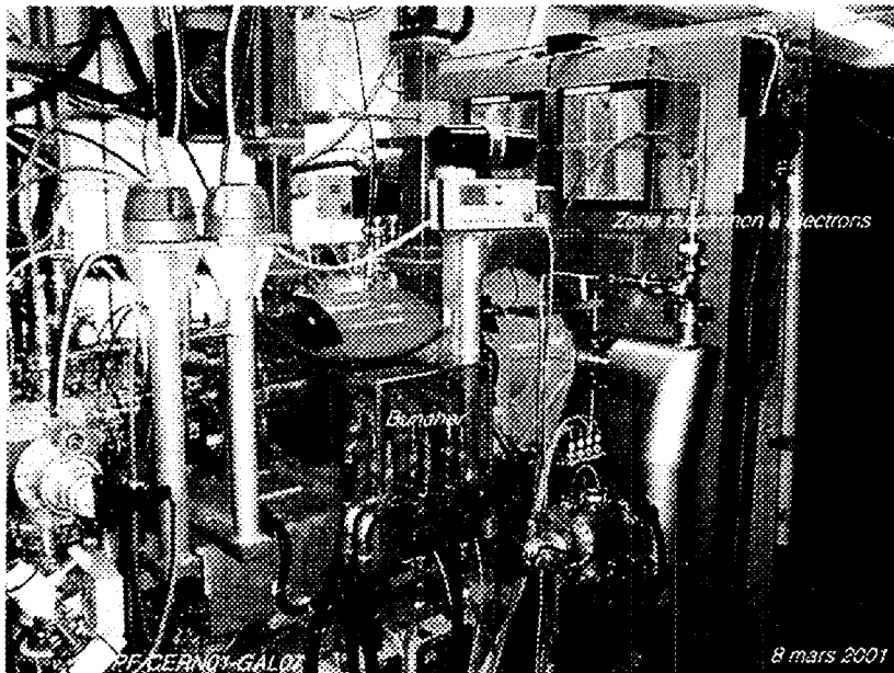
Vue partielle : Le canon ; Le pré-groupeur Le groupeur (buncher).
