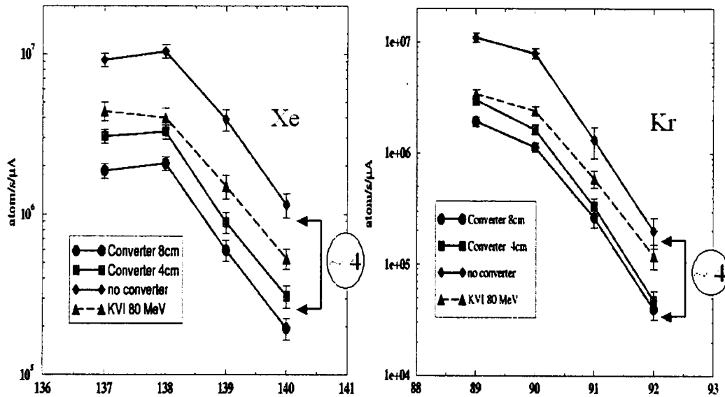
Figure 1 : comparaison de la production d'isotopes de gaz rares obtenue par photo-fission dans différentes configurations (courbes : rouge, verte, bleue) avec celle obtenue au KVI en utilisant un faisceau de deutons de 80 MeV
