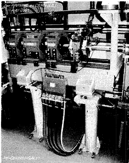
Vue partielle : Le triplet en sortie de section accélératrice
