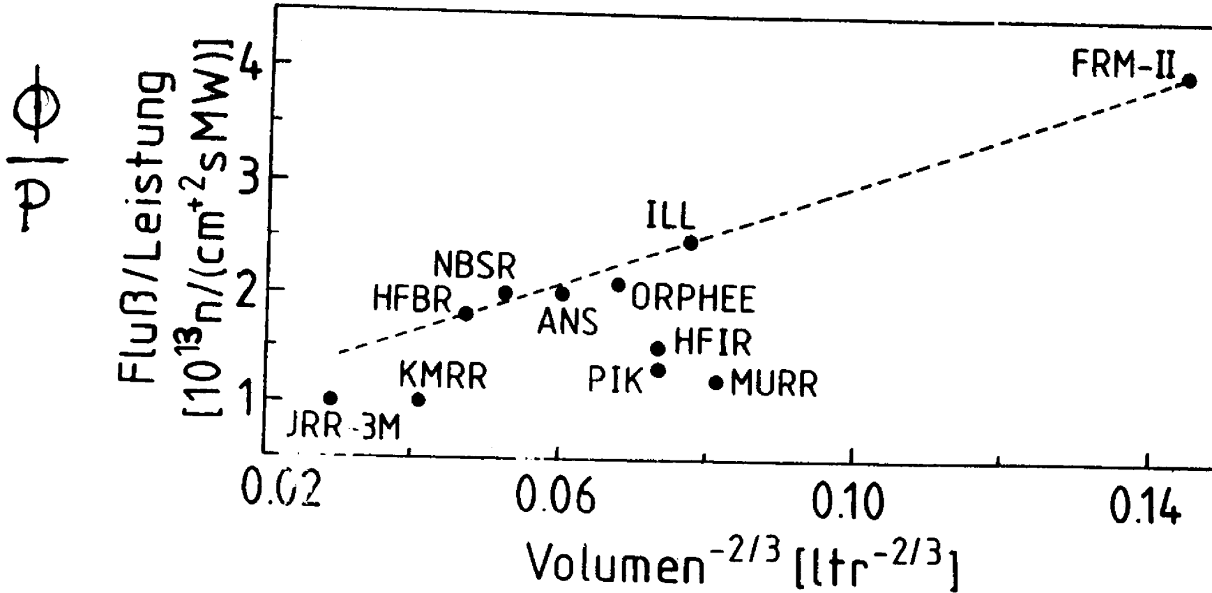
Abb.1: Flußoptimierung verschiedener Neutronenquellen (HFBR: Brookhaven; NBSR: National Institute of Standards and Technology; ANS: Oak Ridge; Orphée: Saclay; ILL: Grenoble).
