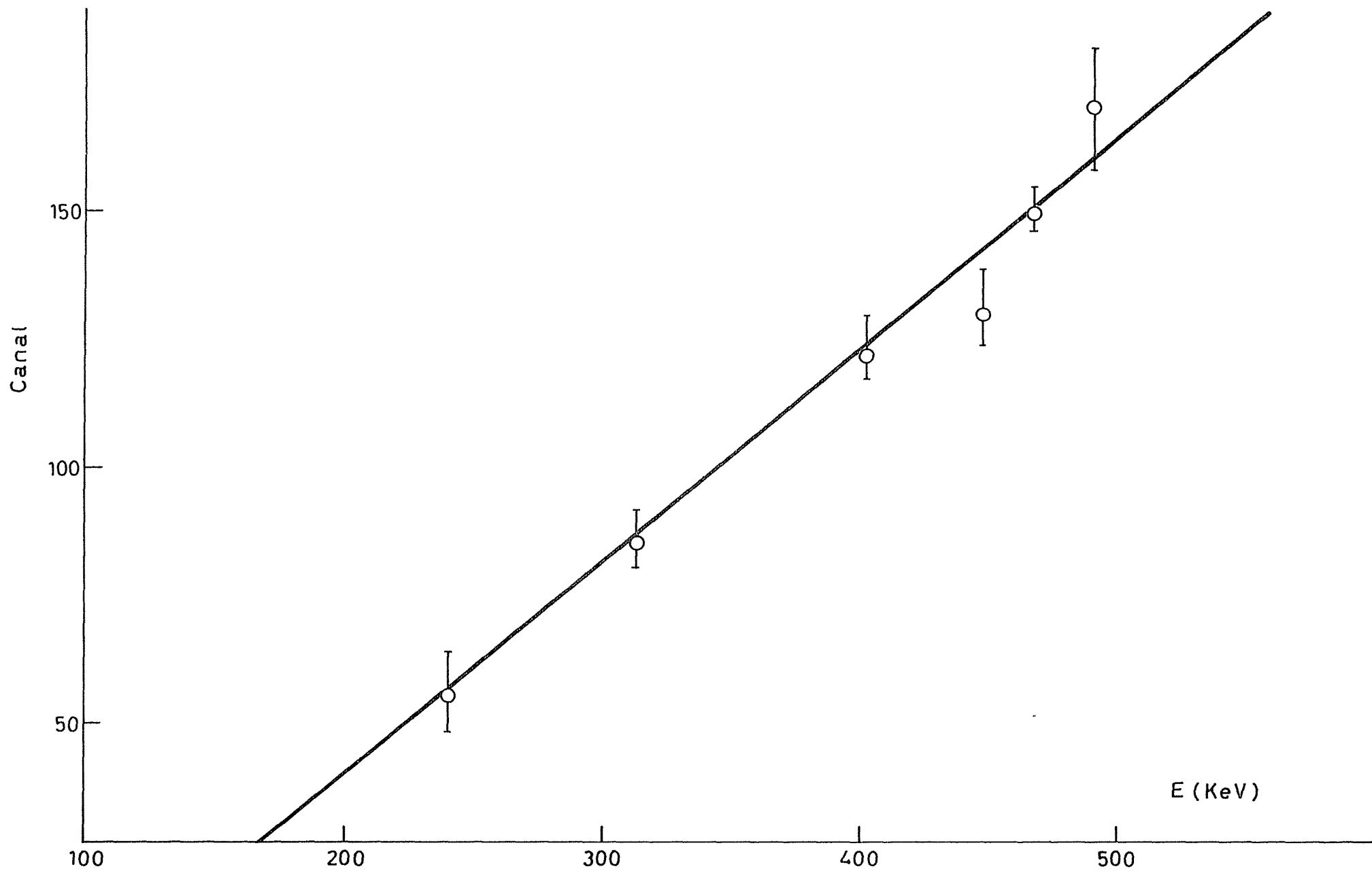
Fig. A4.-Recta de calibración energía - canal
