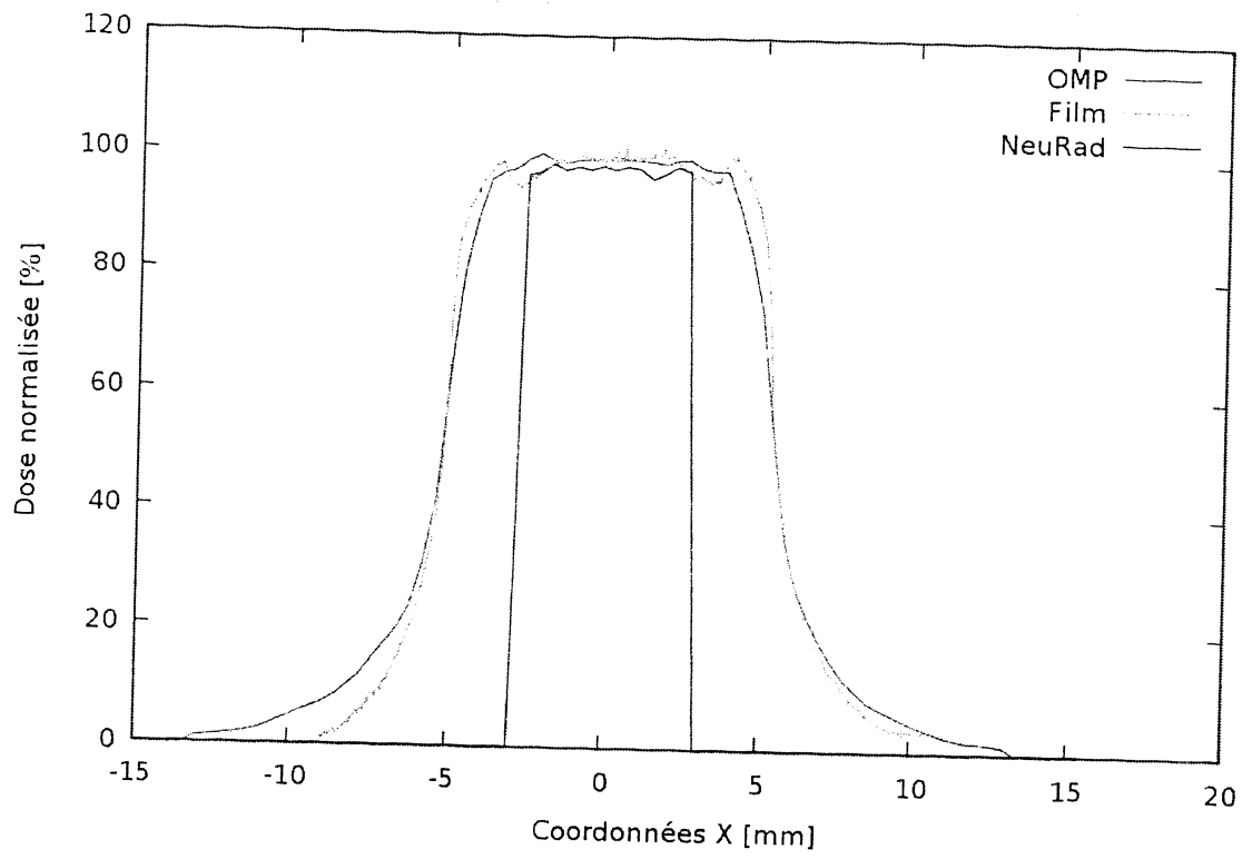
Figure 6 : Profils au centre de l'hétérogénéité (profondeur 155 mm)
