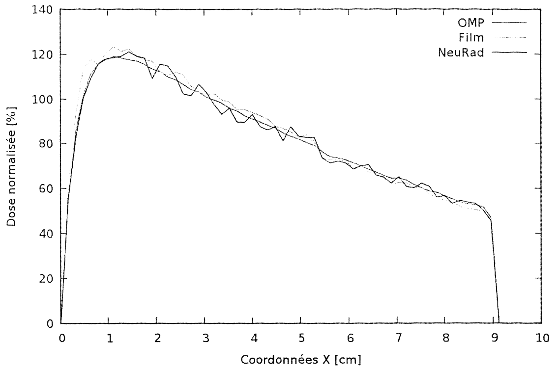
Figure 4 : Rendements en profondeur.
