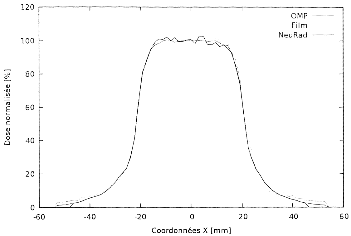
Figure 5 : Comparaison des profils à l'isocentre
