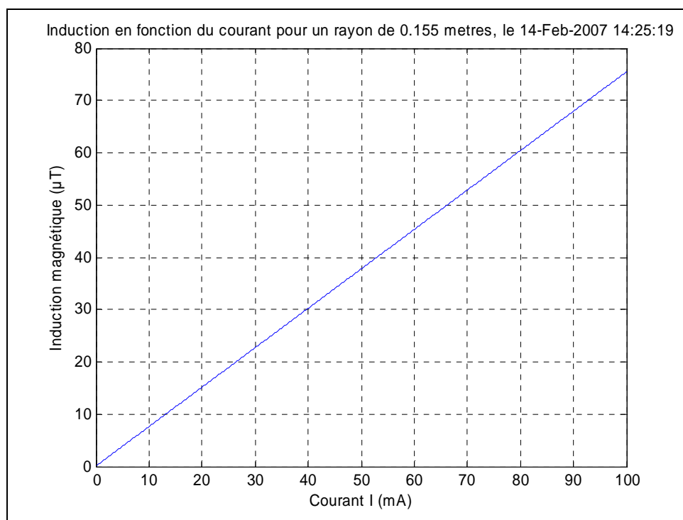
Figure 13 : Relation théorique entre le courant circulant dans les bobines de Helmholtz et l'induction créée sur l'axe au milieu des deux bobines
