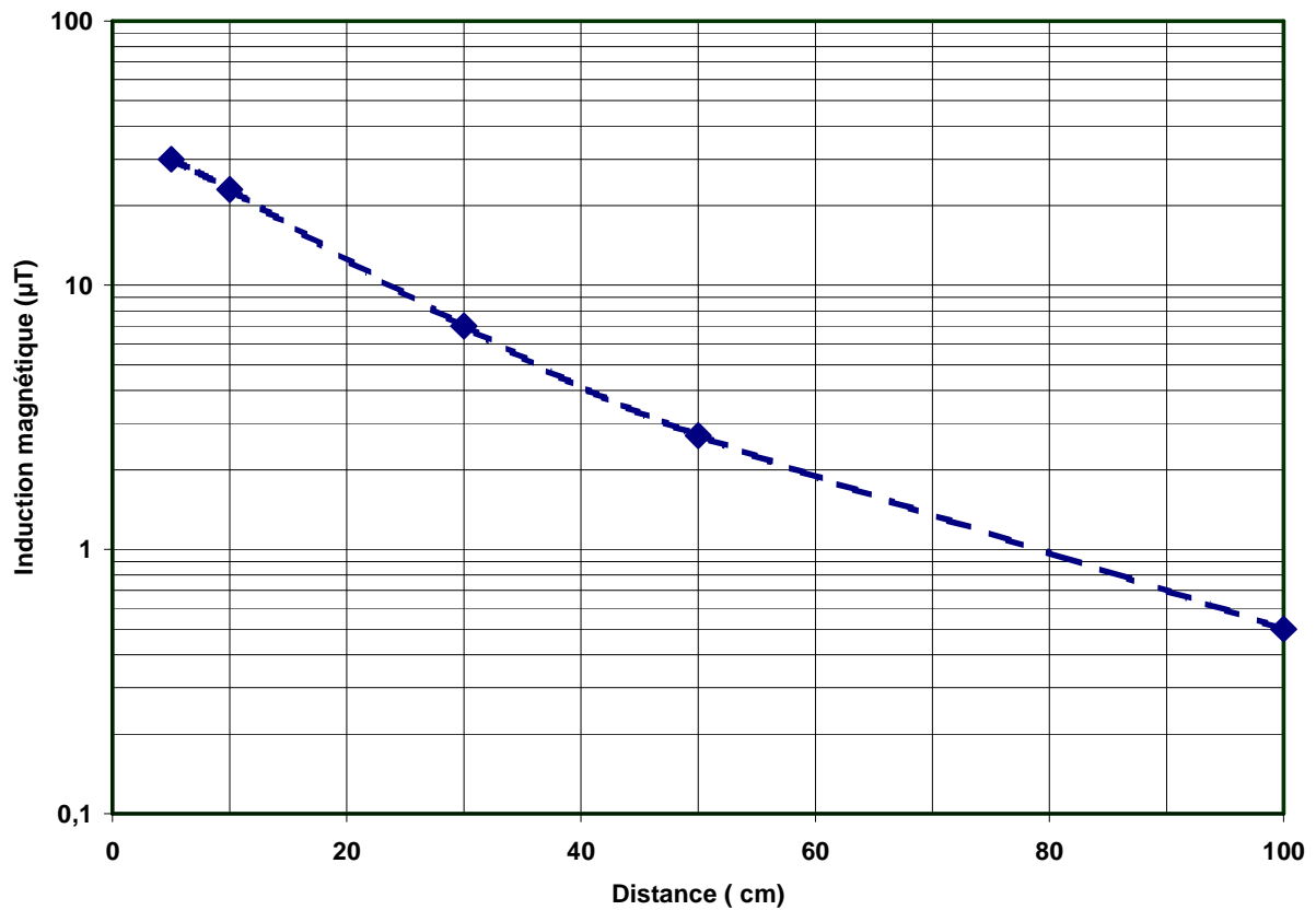
Figure A17 : Variation de l'induction (champ) magnétique avec la distance : Four à micro-ondes M9
