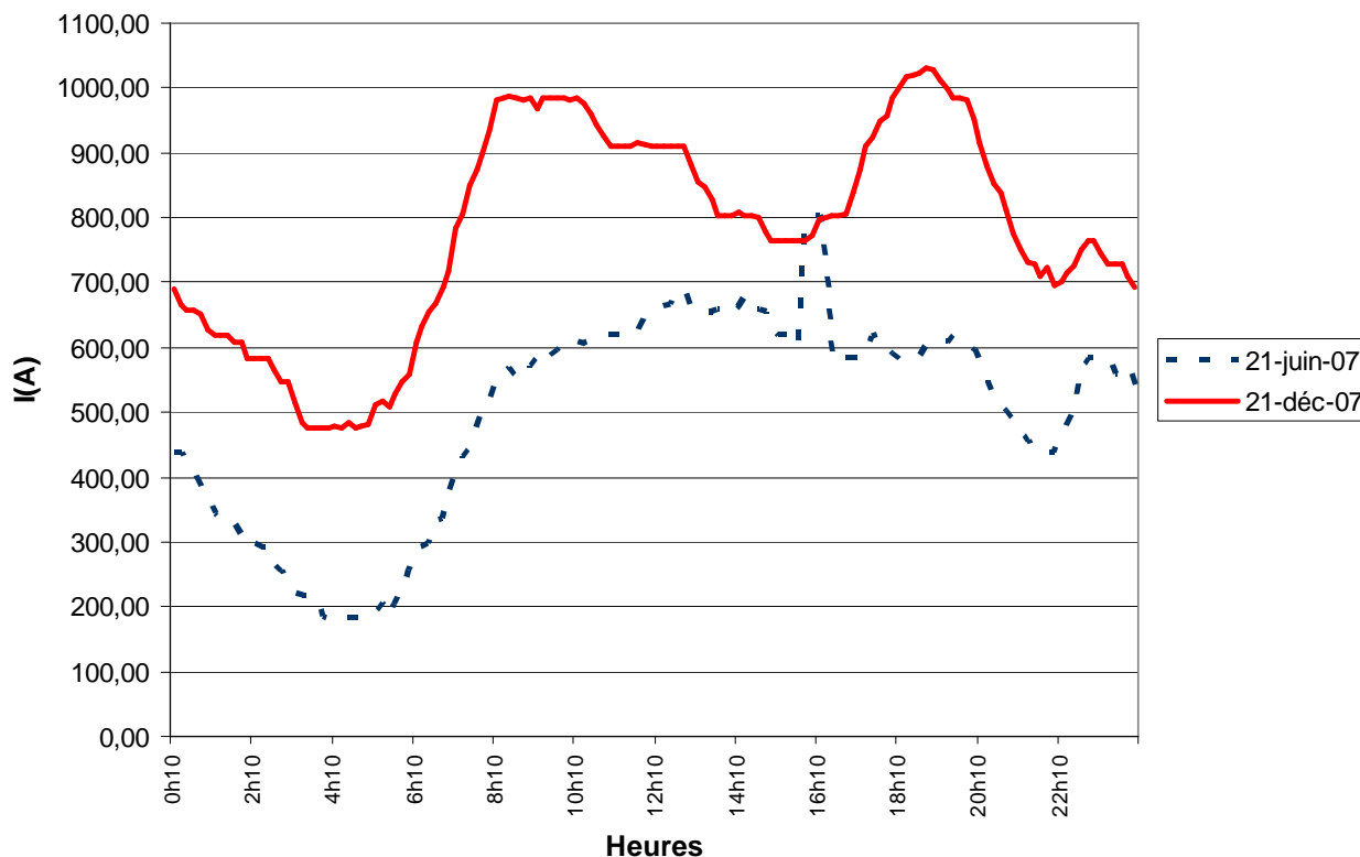
Figure 4 : Évolution de l'intensité du courant sur un type de ligne à 400 kV de la région parisienne. Source : RTE
