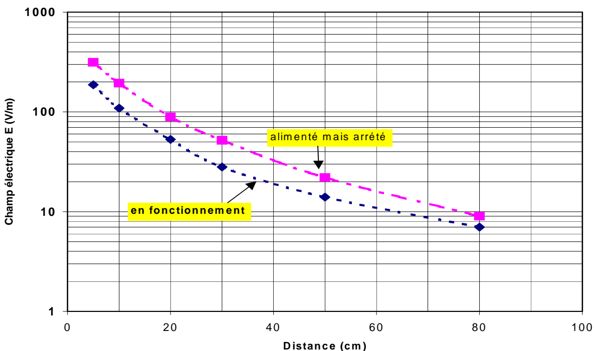
Figure A21 : Variation du champ électrique avec la distance : Sèche-cheveux M11
