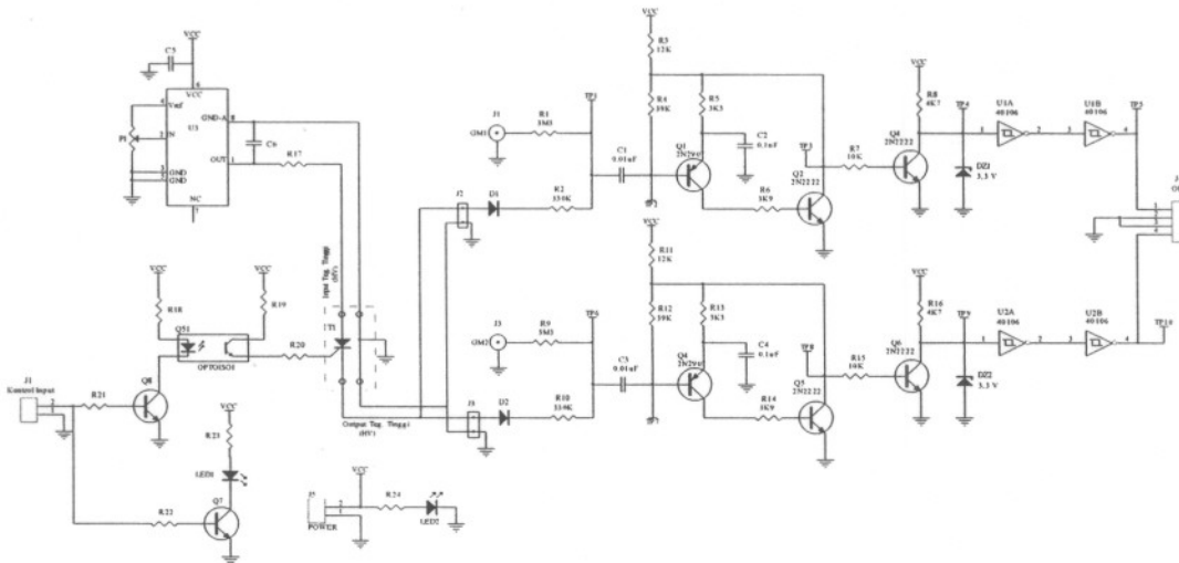
Gambar 6. Rangkaian Skematik Pengolah Sinyal
