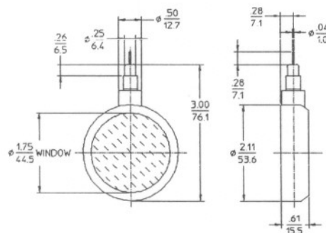
Gambar 4. Detektor GM Type Pancake sebagai Sistem Deteksi [4]
