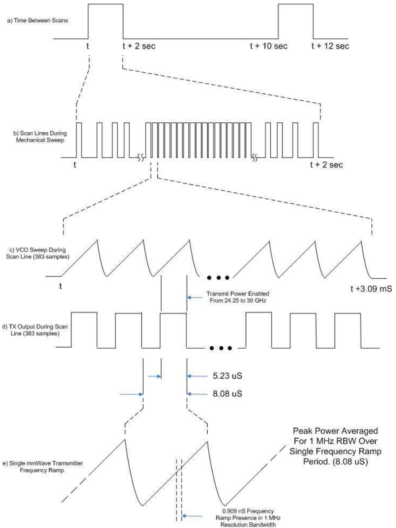
Figure 4 : Représentation schématique d'un cycle de fonctionnement d'un scanner corporel
