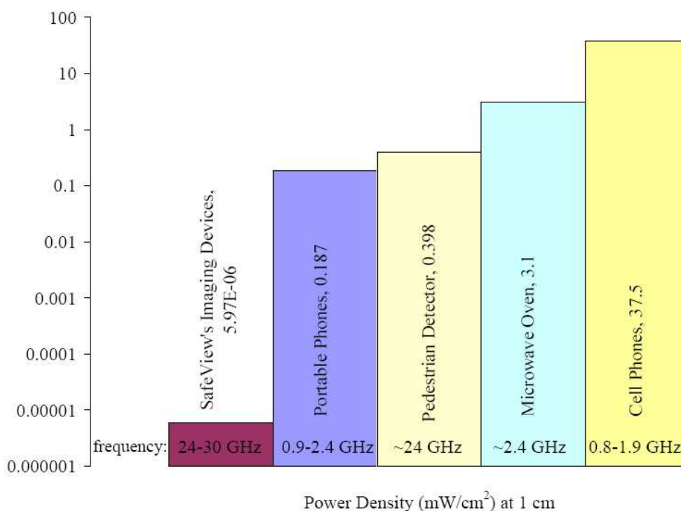
Figure 9 : Comparaison des densités de puissance (mW/cm 2 ) émises (mesurées à 1 cm) par différents appareils de consommation courants et un scanner corporel à ondes « millimétriques »
