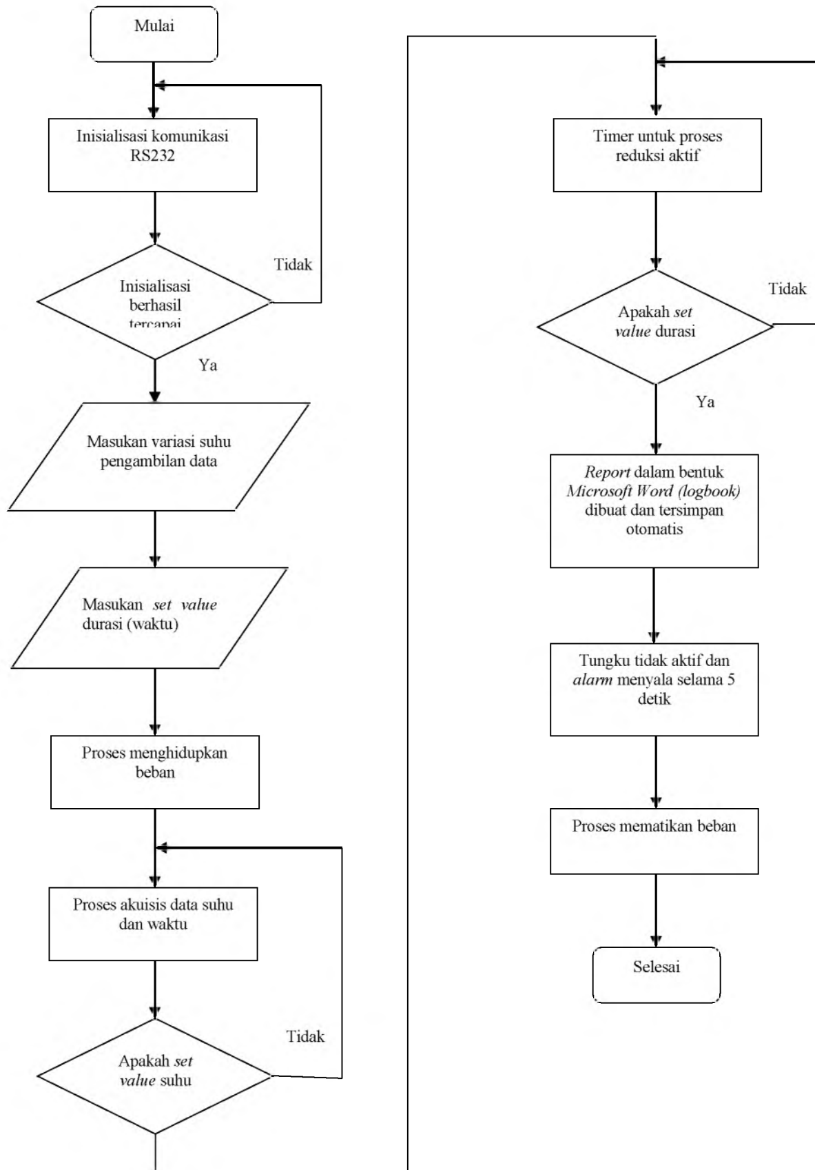
Gambar 5. Diagram alir sistem secara keseluruhan
