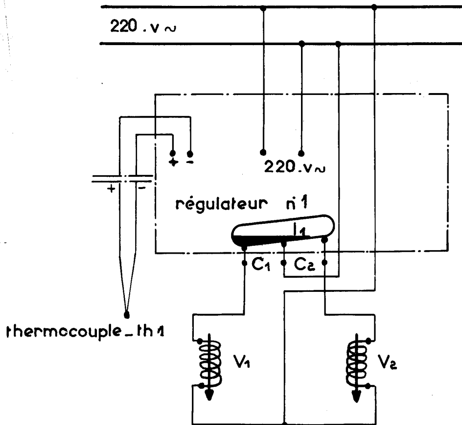
FIG. 2 - SCHEMA ELECTRIQUE
