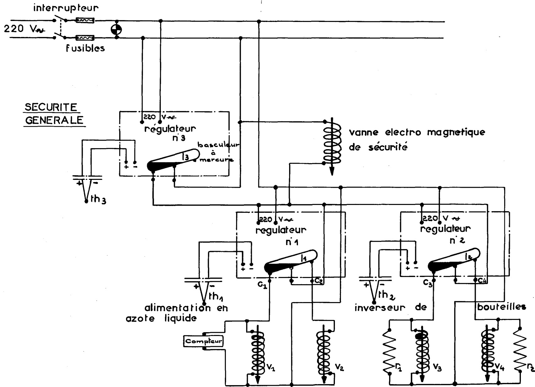
FIG. 6 - SCHEMA ELECTRIQUE
