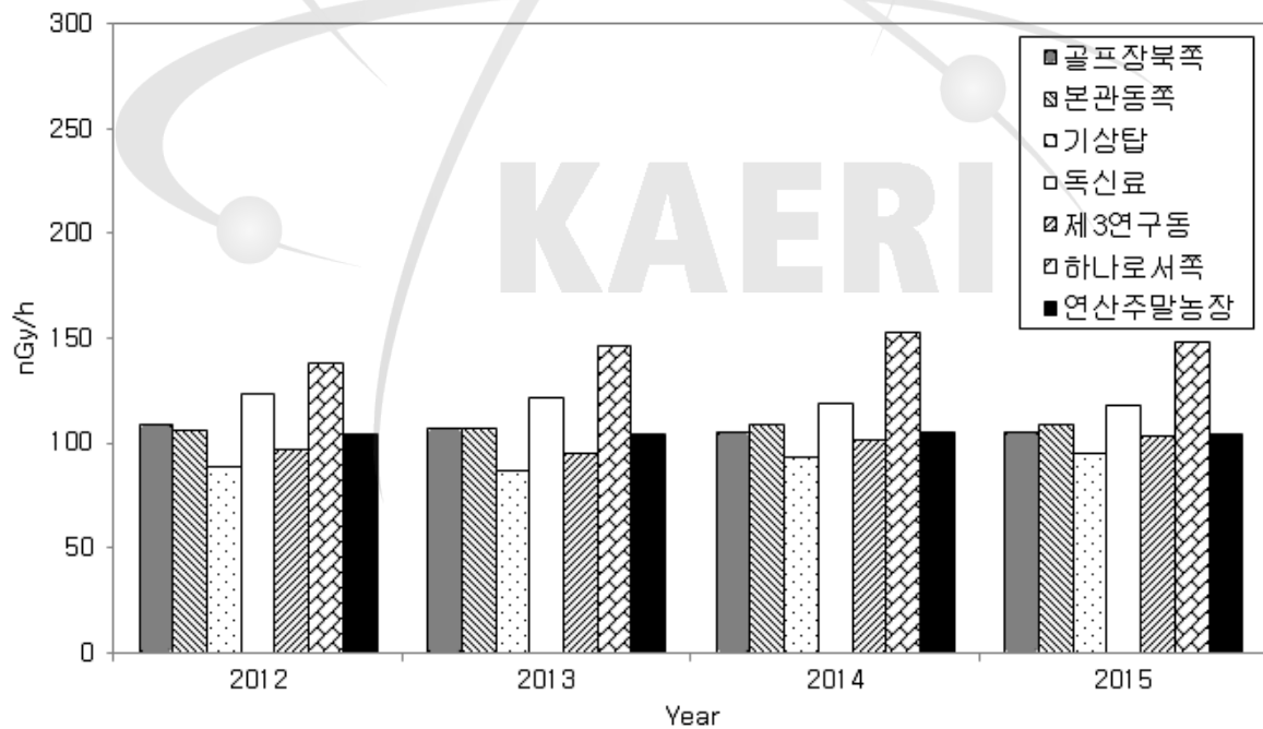
그림 2-9. 대덕 원자력시설 주변 공간감마선량률 (환경방사선감시기)
