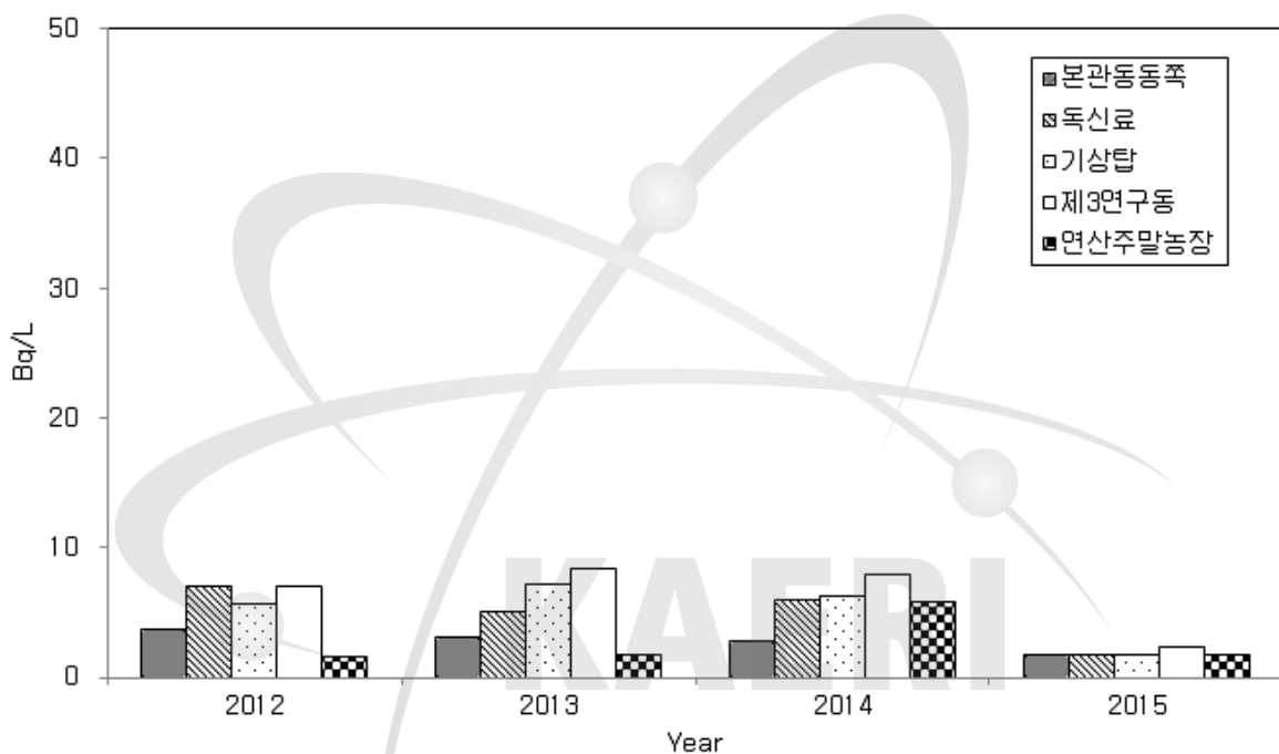
그림 2-18. 대덕 원자력시설 주변 빗물의 방사능 농도 (삼중수소)
