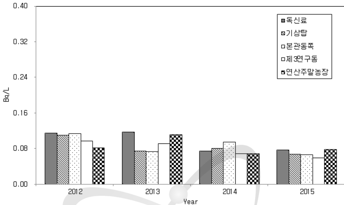
그림 2-19. 대덕 원자력시설 주변 빗물의 방사능 농도 (전베타)
