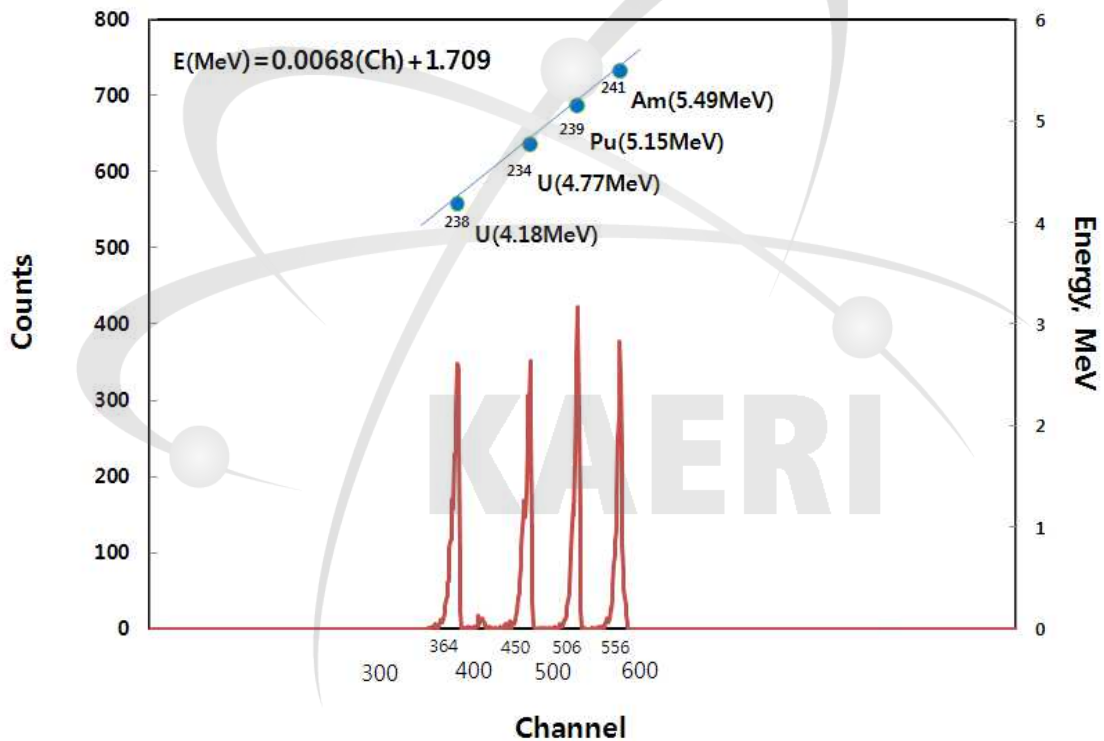
그림 2-8. 알파 스펙트로메타의 에너지 보정 곡선
