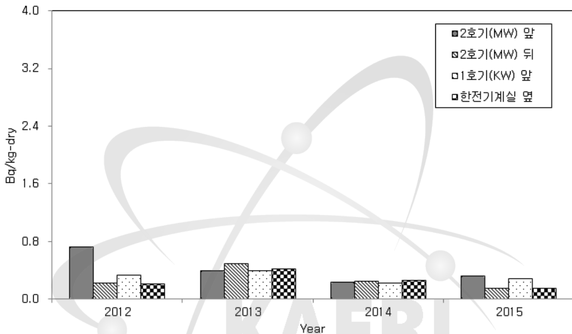
그림 2-28. TRIGA 연구로 시설 주변 토양의 방사능 농도 (스트론튬-90)
