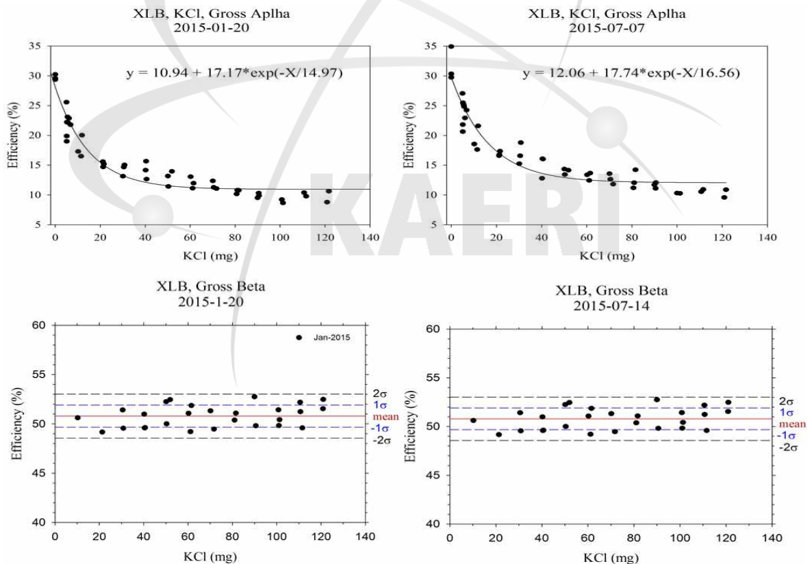
그림 2-6. 저준위 알파/베타계수기 자기흡수 보정 결과
