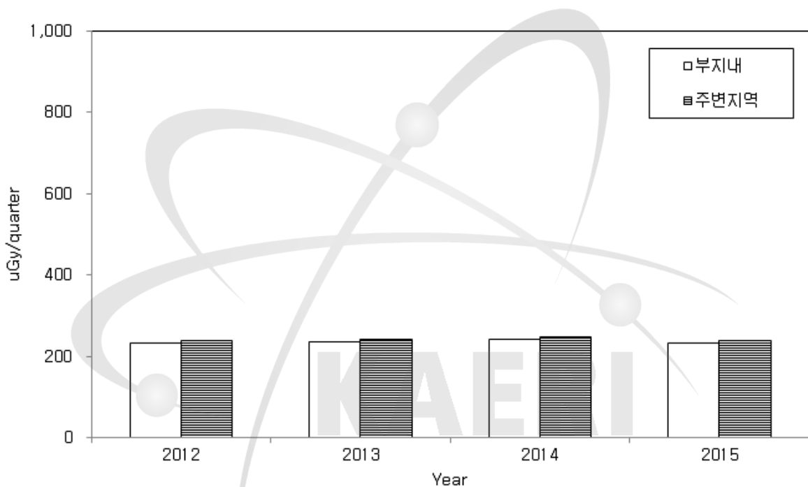
그림 2-26. TRIGA 연구로시설 주변 공간집적선량 (열형광선량계)
