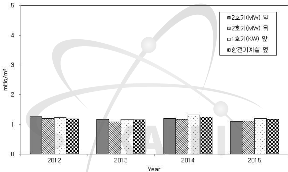
그림 2-27. TRIGA 연구로시설 주변 공기 중 미립자의 방사능 농도 (전베타)
