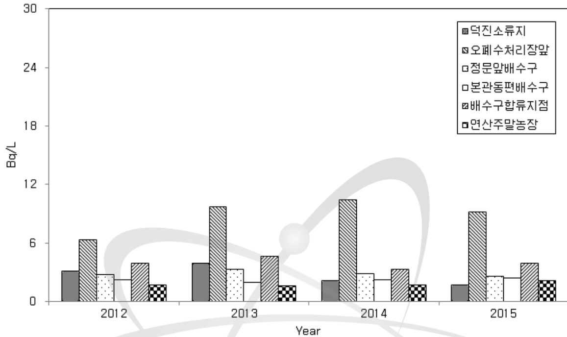
그림 2-20. 대덕 원자력시설 주변 지표수의 방사능 농도 (삼중수소)
