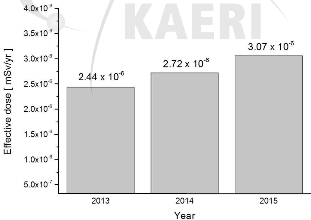
그림 4-2. 최근 3년간 액체상 방출물에 의한 부지 최대 피폭연령군의 유효선량
