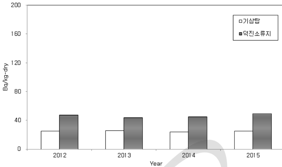
그림 2-15. 대덕 원자력시설 주변 토양의 방사능 농도 ( ^{238}\text{U} )
