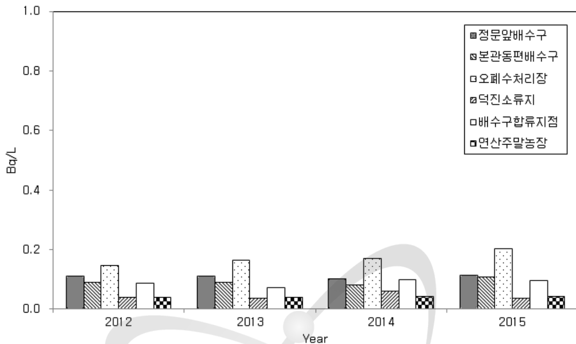
그림 2-21. 대덕 원자력시설 주변 지표수의 방사능 농도 (전베타)
