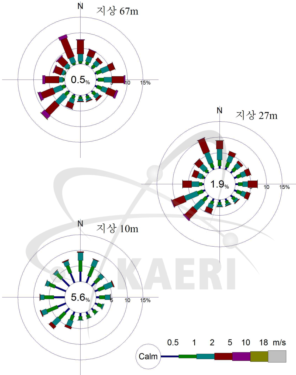
그림 3-1 연간 바람장미(Annual wind rose) (동심원내 숫자는 정온상태 발생빈도의 백분율을 나타냄)
