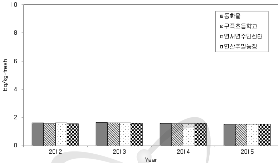
그림 2-24. 대덕 원자력시설 주변 농산물(배추)의 방사능 농도 (삼중수소)
