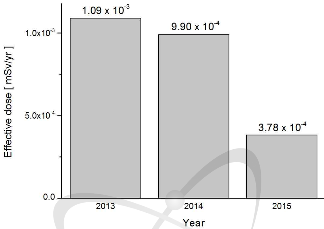
그림 4-1. 최근 3년간 기체상 방출물에 의한 부지 최대 피폭연령군의 유효선량
