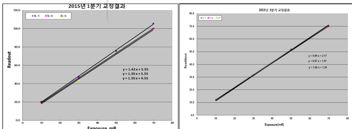
그림 2-7. TLD Reader 보정 결과
