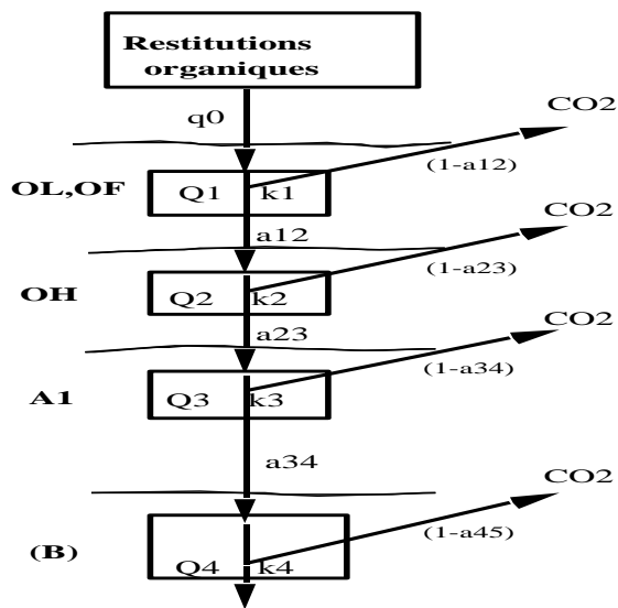
Figure : (a) Compartiments et flux dans un sol forestier et (b) détail pour un horizon
