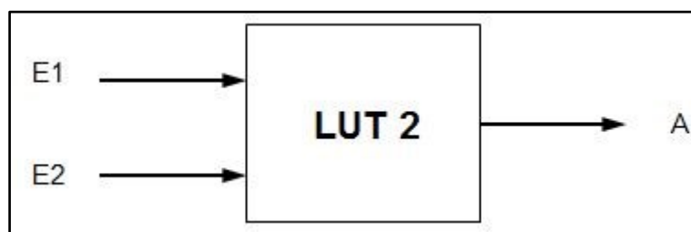
Bild 6.2: Look-Up Table
