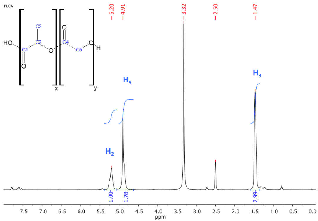
Figura 3.14 – Espectro de RMN ^1\text{H} do PLGA em DMSO, 400 MHz.
