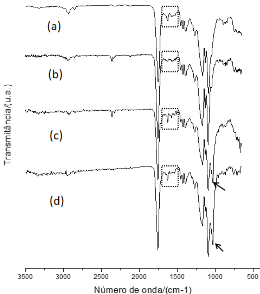
Figura 3.27 – Espectros de ATR-FTIR das nanofibras com matrizes de PLGA-S: (a) PLGA-S; (b) PLGA-S/MCC; (c) PLGA-S/HAm e (d) PLGA-S/HAm/MCC. As setas indicam a presença da banda referente ao estiramento P-O da n-HAm e os quadrados pontilhados mostram a presença de bandas características do ligante SMZ.
