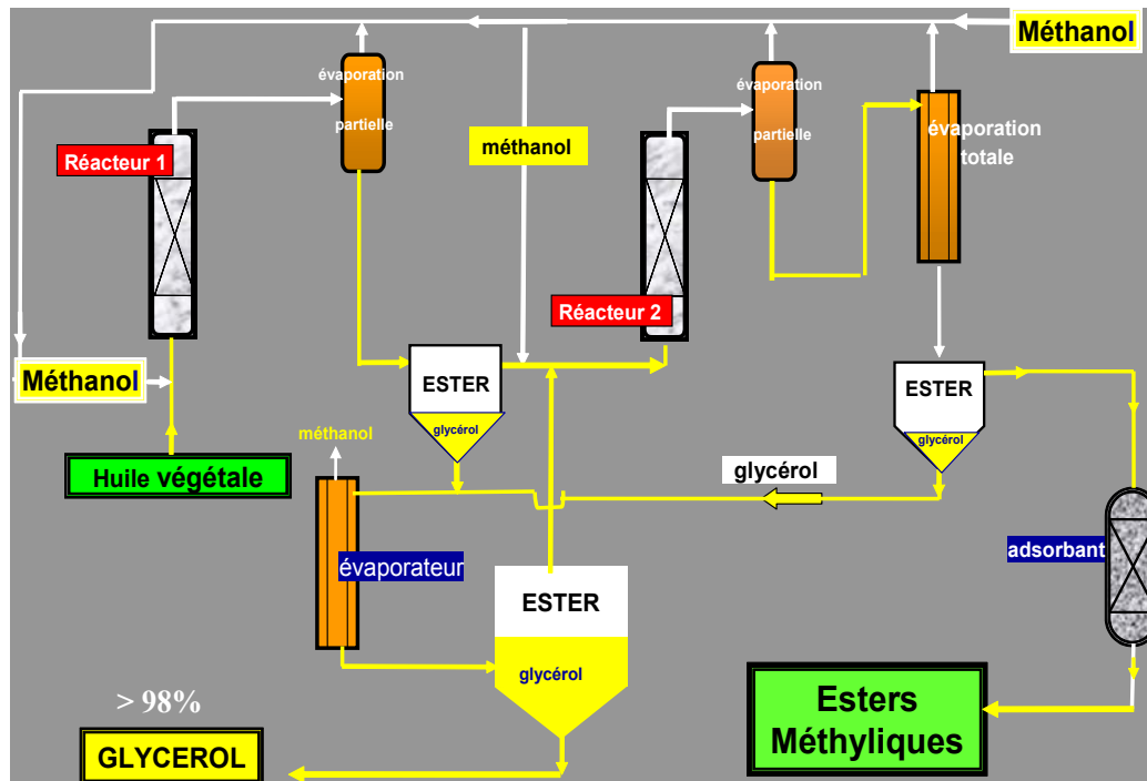
Schéma 2 - Schéma de principe du procédé Esterfip Hétérogène
