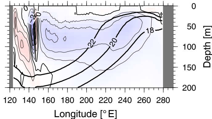
(b) W reg. Nino3, OLD
