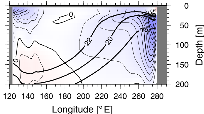
(d) DIC reg. Nino3, OLD
