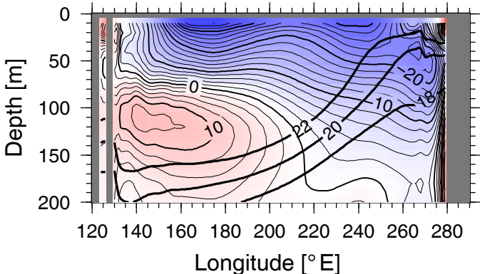
(c) DIC reg. Nino3, NEW
