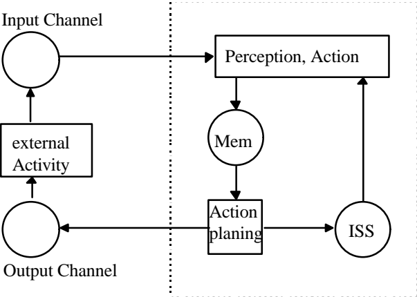
Abbildung 3: Wahrnehmung und Komplexität, aus [Rauterberg 1995]
