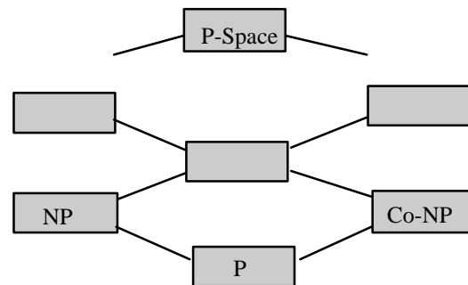
Abbildung 1: Polynomiale Hierarchie
