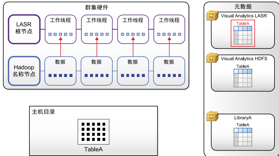
图 5.4 从并置存储加载
