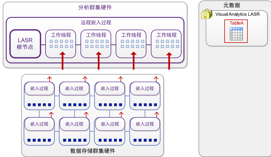
图 5.5 使用 SAS Embedded Process 导入
