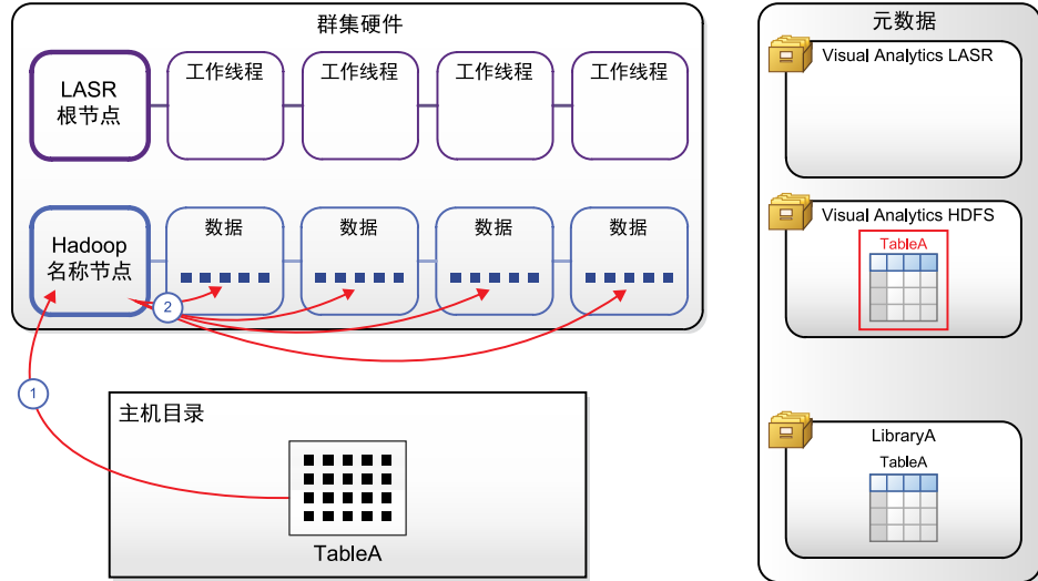
图 5.4 从并置存储加载
