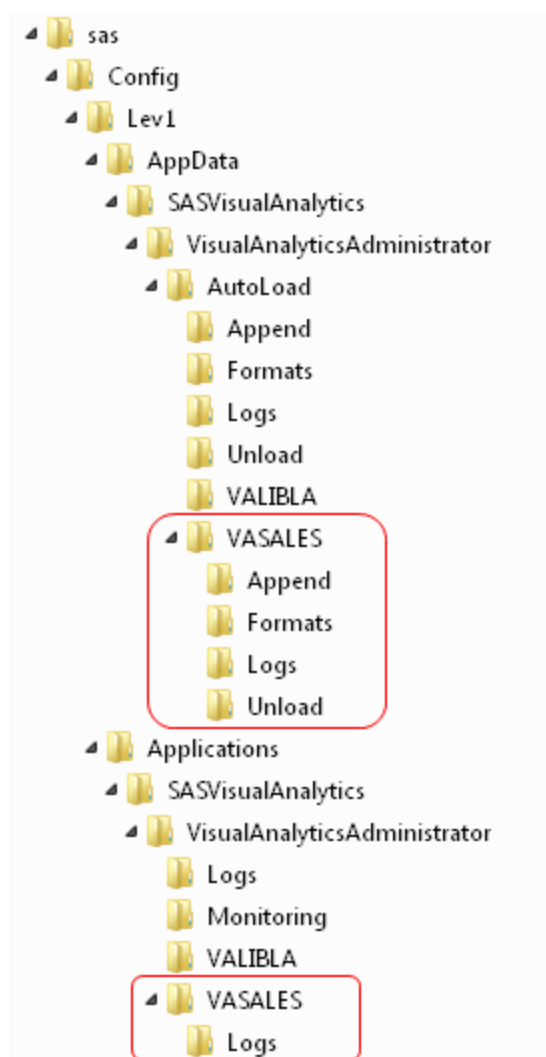
图 2.1 示例：自动加载的 VASALES 实现
