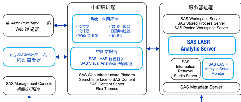
图 A1.1 客户端、中间层和服务器
