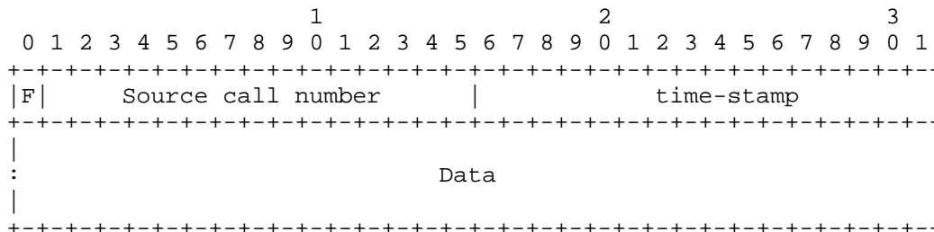
Figure 6: Mini Frame Binary Format
