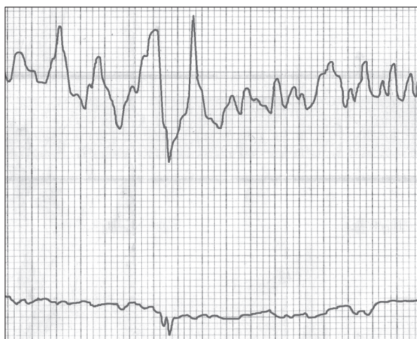
Рис. 3. Участок спектра поглощения (центр – 3300 Гс, диапазон – 400 Гс) образца \text{NH}_4\text{I} после трех актов нагружения: вверху – параллельная, внизу – перпендикулярная ориентация образца в форме диска в магнитном поле.
