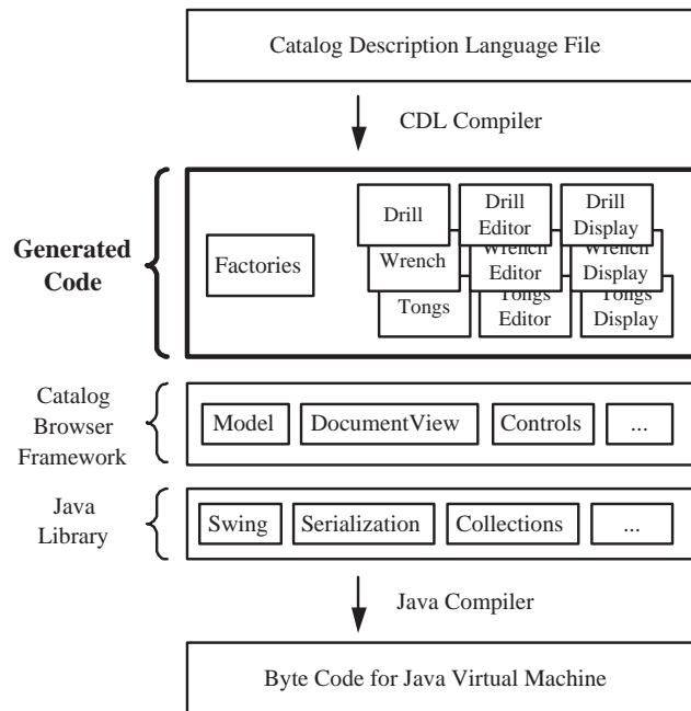
Fig. 6. CDL stack
