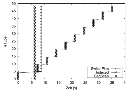
(b) Nested Loops auf part ⋈ partsupp
